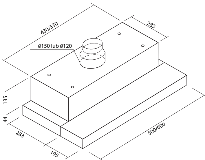
Okap VEGA/VEGA GLASS
